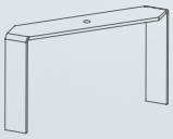
Sıva Altı Montaj Parçası / Recessed Mounting Piece
